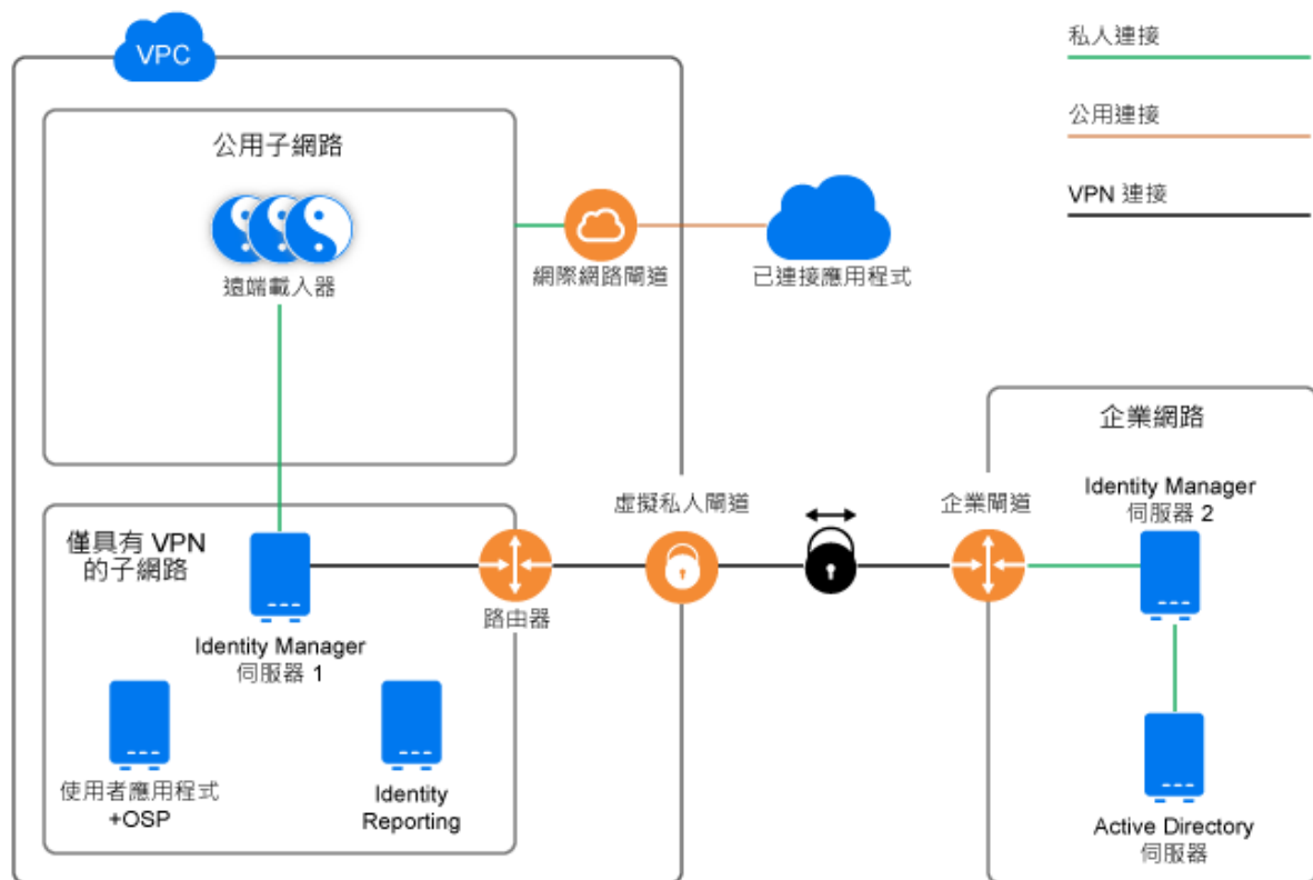
圖 15-2 使用多伺服器驅動程式集連接的混合式方案
