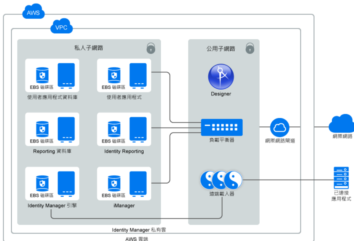
圖 14-1 AWS EC2 上的 Identity Manager 部署
