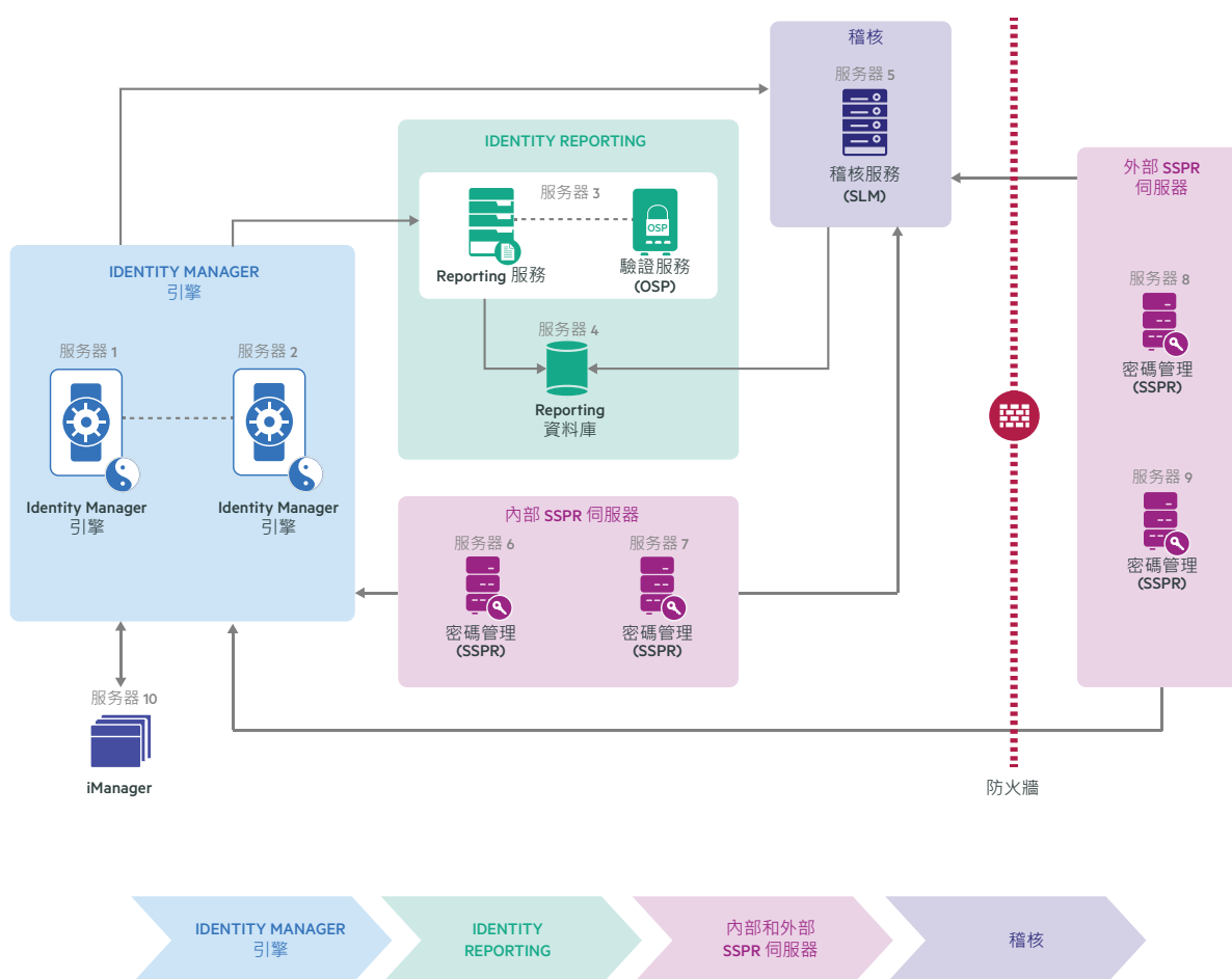
圖 1-5 範例標準版部署
