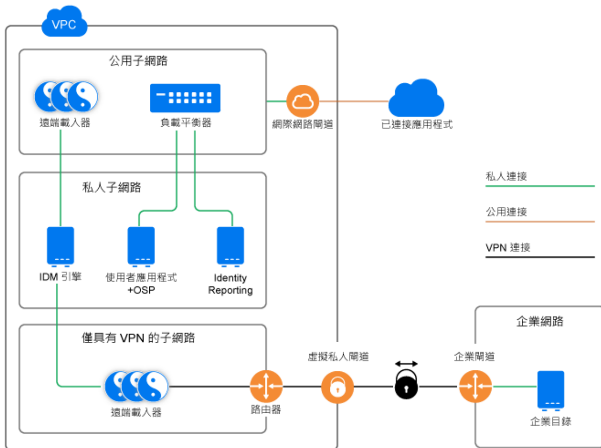
圖 15-1 使用遠端載入器連接的混合式方案
