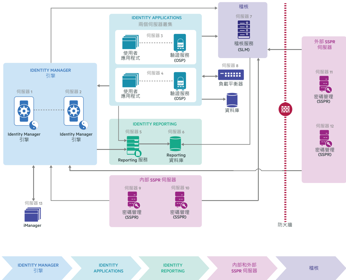
圖 1-4 範例進階版部署
