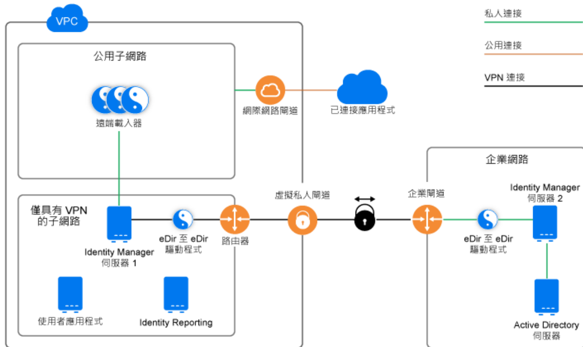
圖 15-4 使用 eDirectory 驅動程式連接的混合式方案
