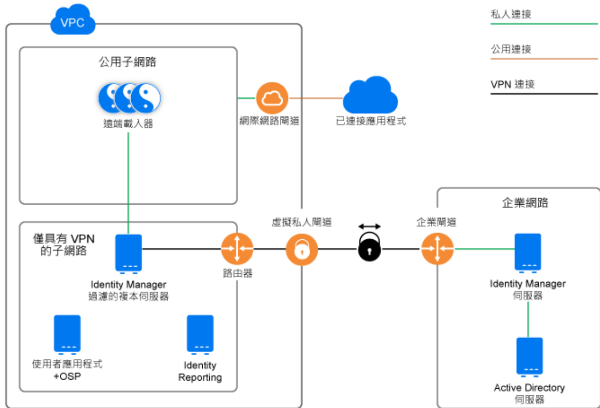
圖 15-3 使用受控複製的混合式方案
