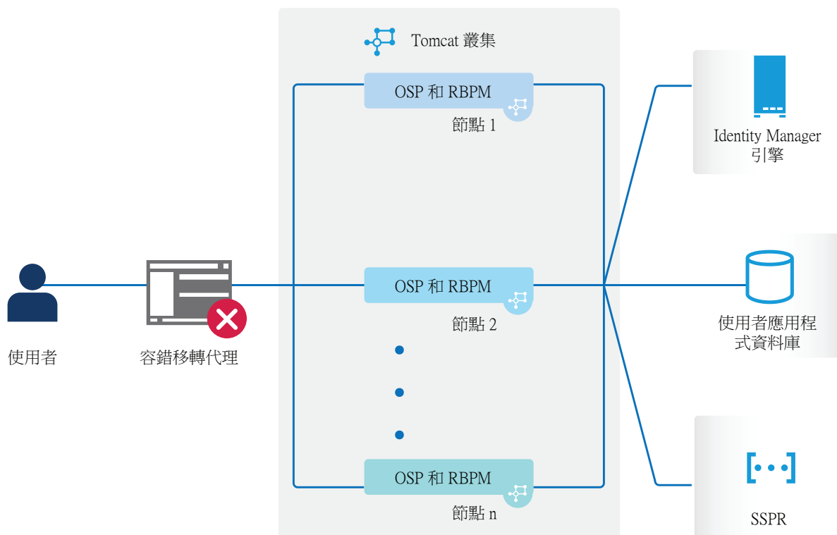
圖 18-1 叢集部署解決方案範例
